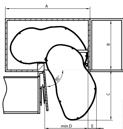
Установка стеллажа на боковую часть корпуса
