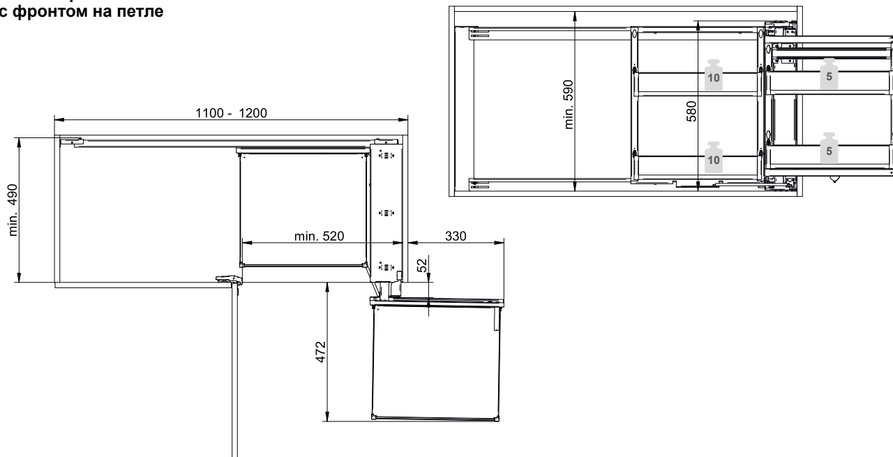
Corner Space 1100 - 1200 с фронтом на петле
